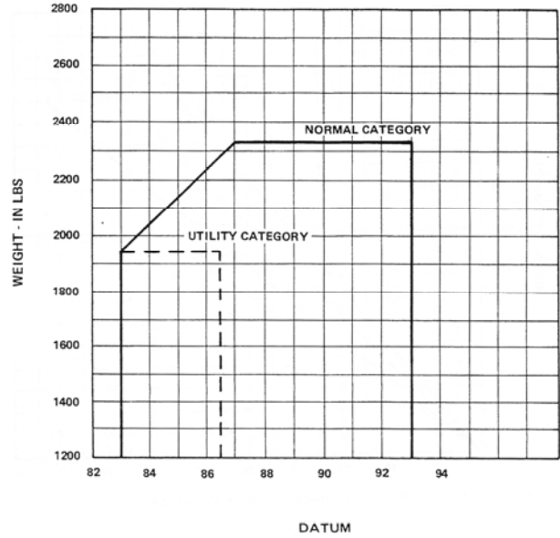
C. G. RANGE AND WEIGHT
